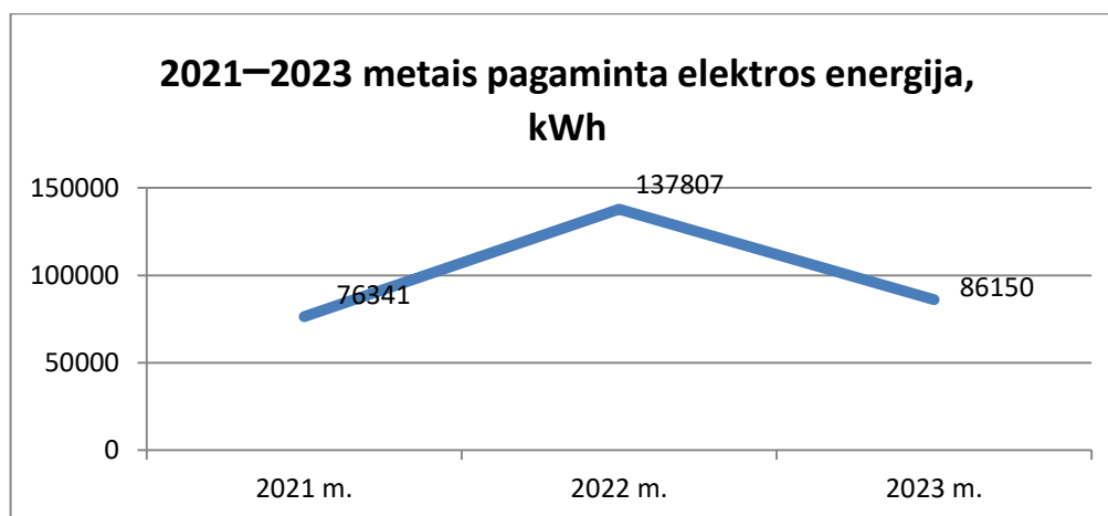
17 pav. 2021–2023 m. pagaminta elektros energija, kWh
